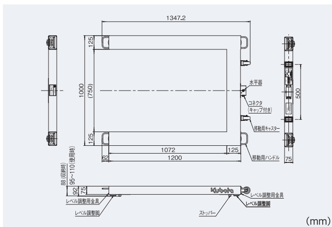
正確な計量を保証する レベルアジャスター (最薄95mm~)
